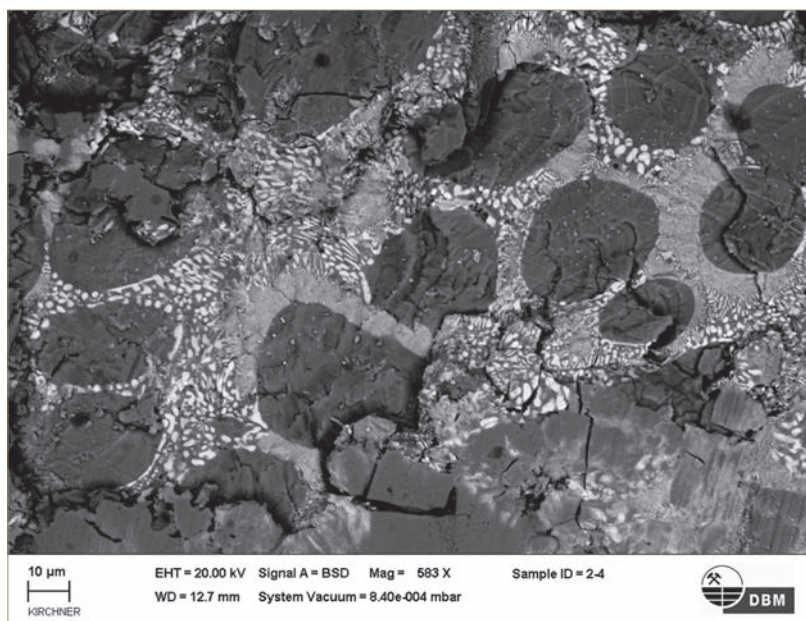
Abb. 5 Beispiel einer Schlackenprobe mit inhomogenem Gefüge. Die hellen, tupfenartigen Partien bestehen überwiegend aus Blei, während die dunkelgrauen Bereiche neben Blei auch hohe Gehalte von Kupfer und Schwefel aufweisen (Grafik: Deutsches Bergbau-Museum Bochum/D. Kirchner).
